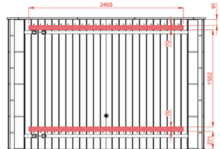
VUE DU DESSOUS
